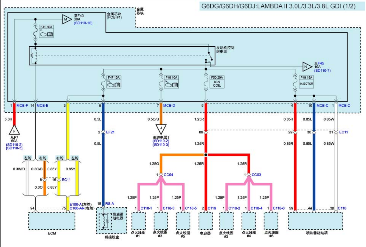
电源分布(6)
